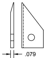
IVB-20 INSERT
